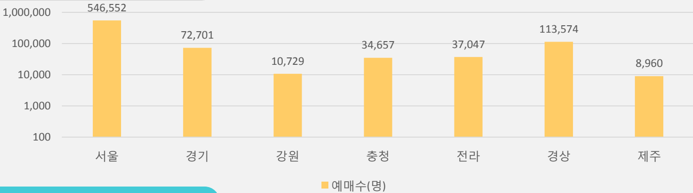
그림 8. 지역별 매출액
