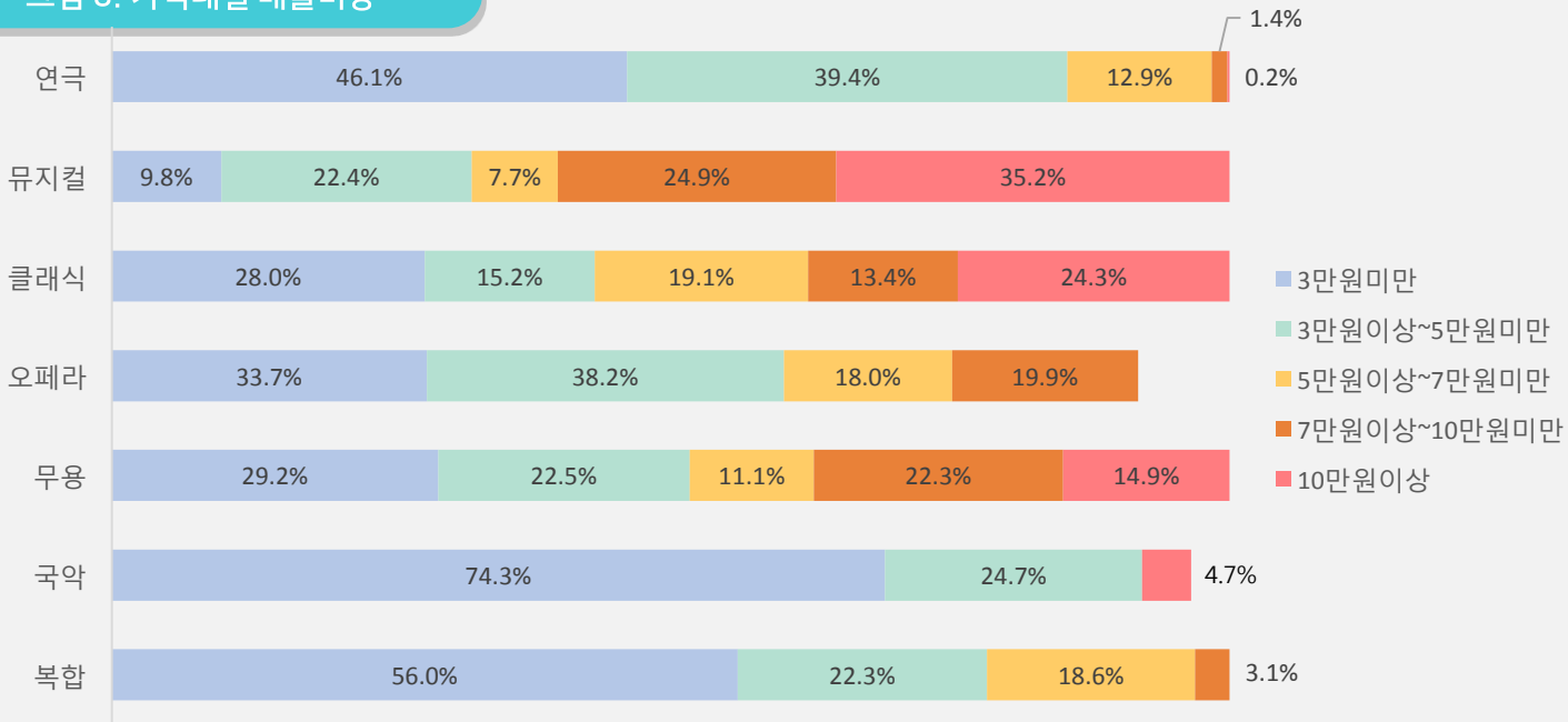
그림 8. 가격대별 매출비중
