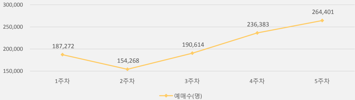
그림 6. 주차별 매출액
