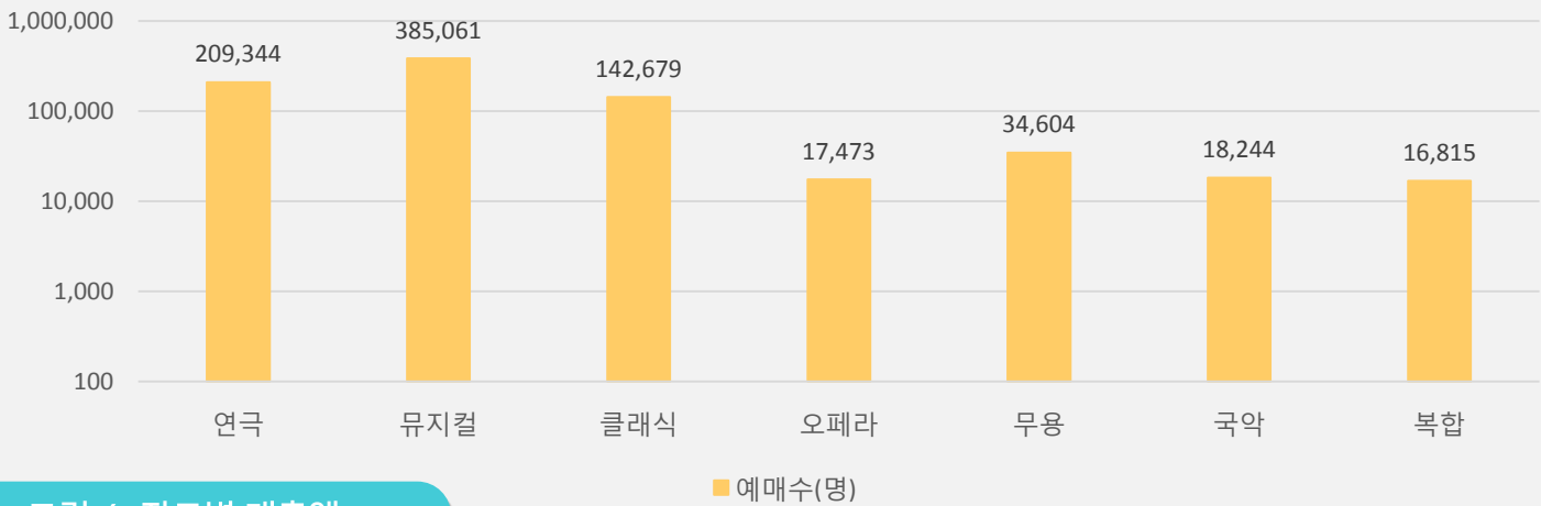
그림 4. 장르별 매출액
